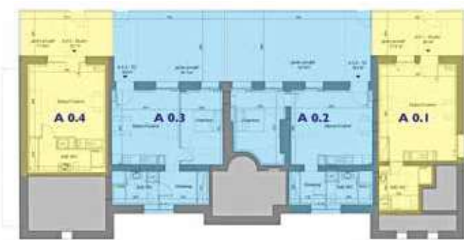
REZ-DE-JARDIN
